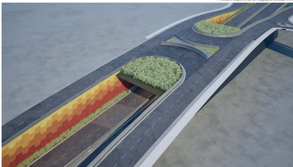
Perspectiva Retorno: Em vez de todos os motoristas compartilharem o mesmo cruzamento para acessar os diferentes sentidos da via, parte dos deslocamentos passa a ser feita por uma estrutura em nível diferente da pista principal
